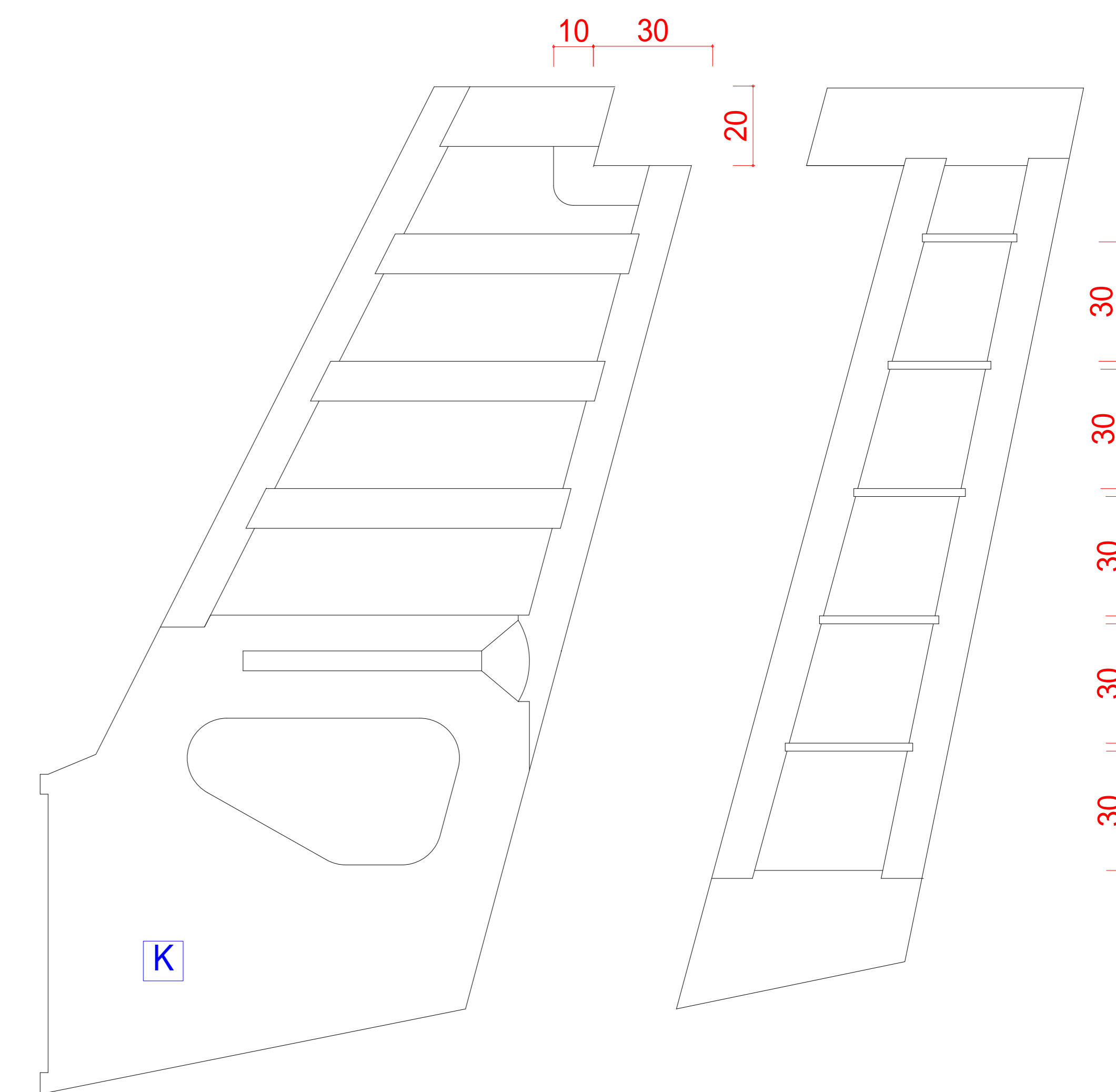
垂直尾翼
