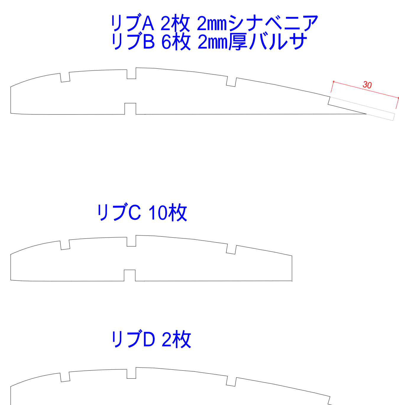
リブ断面図
