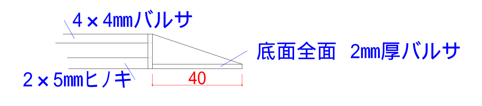
翼端断面
