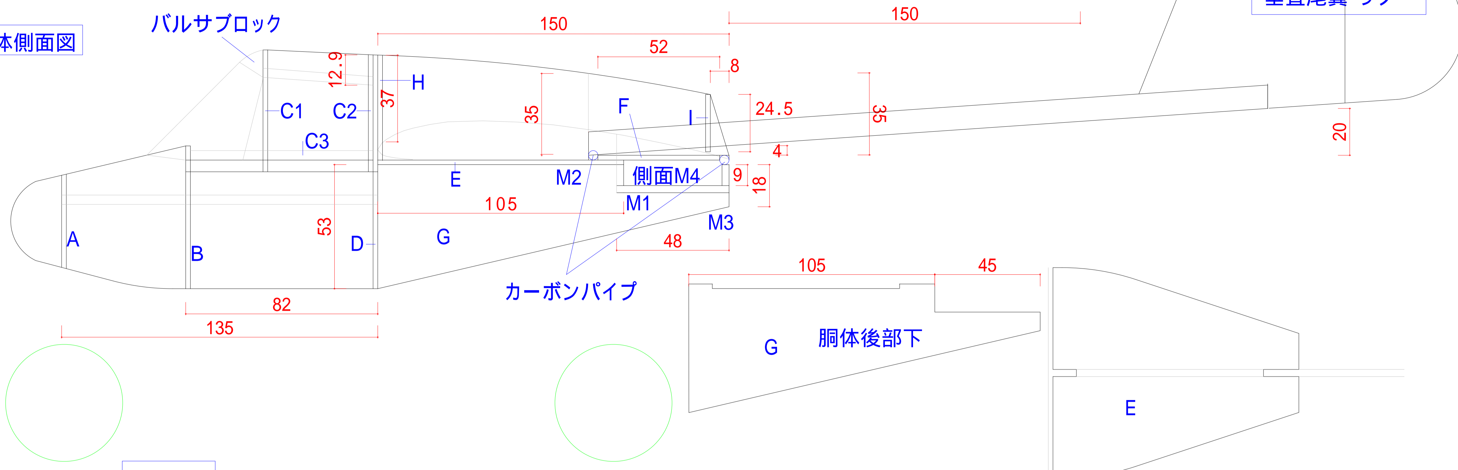
胴体枠
